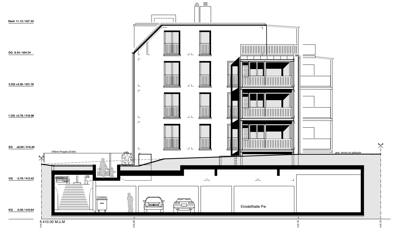
Ansicht Nord - West Haus 6
