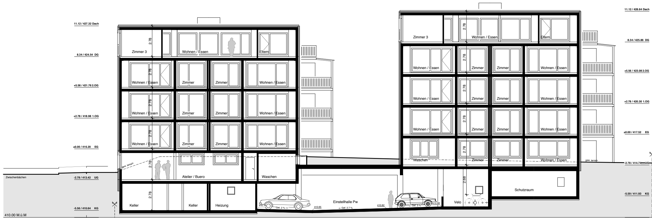
Längsschnitt
